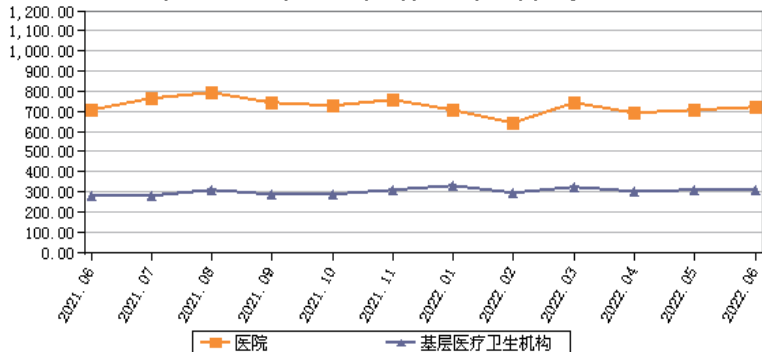
2021年6月-2022年6月全市医疗卫生机构门急诊人次数
